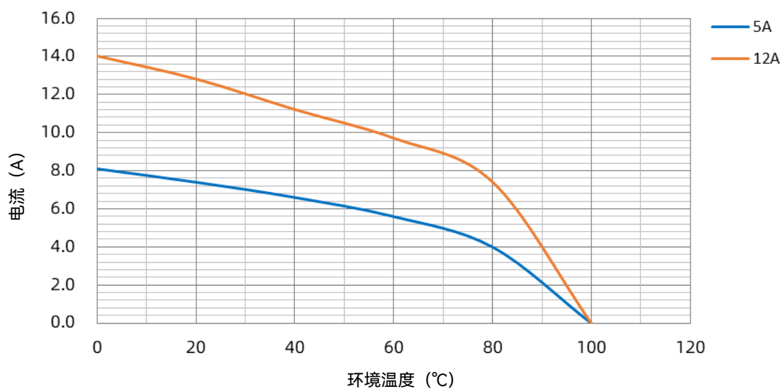
SHG 载流能力曲线
