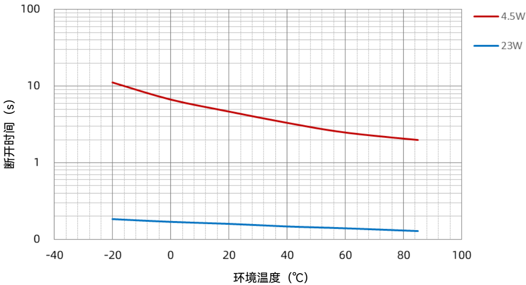
SHG 12 A 功率-温度曲线
