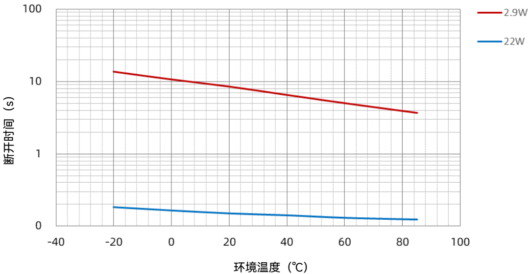
SHG 05 A 功率-温度曲线
